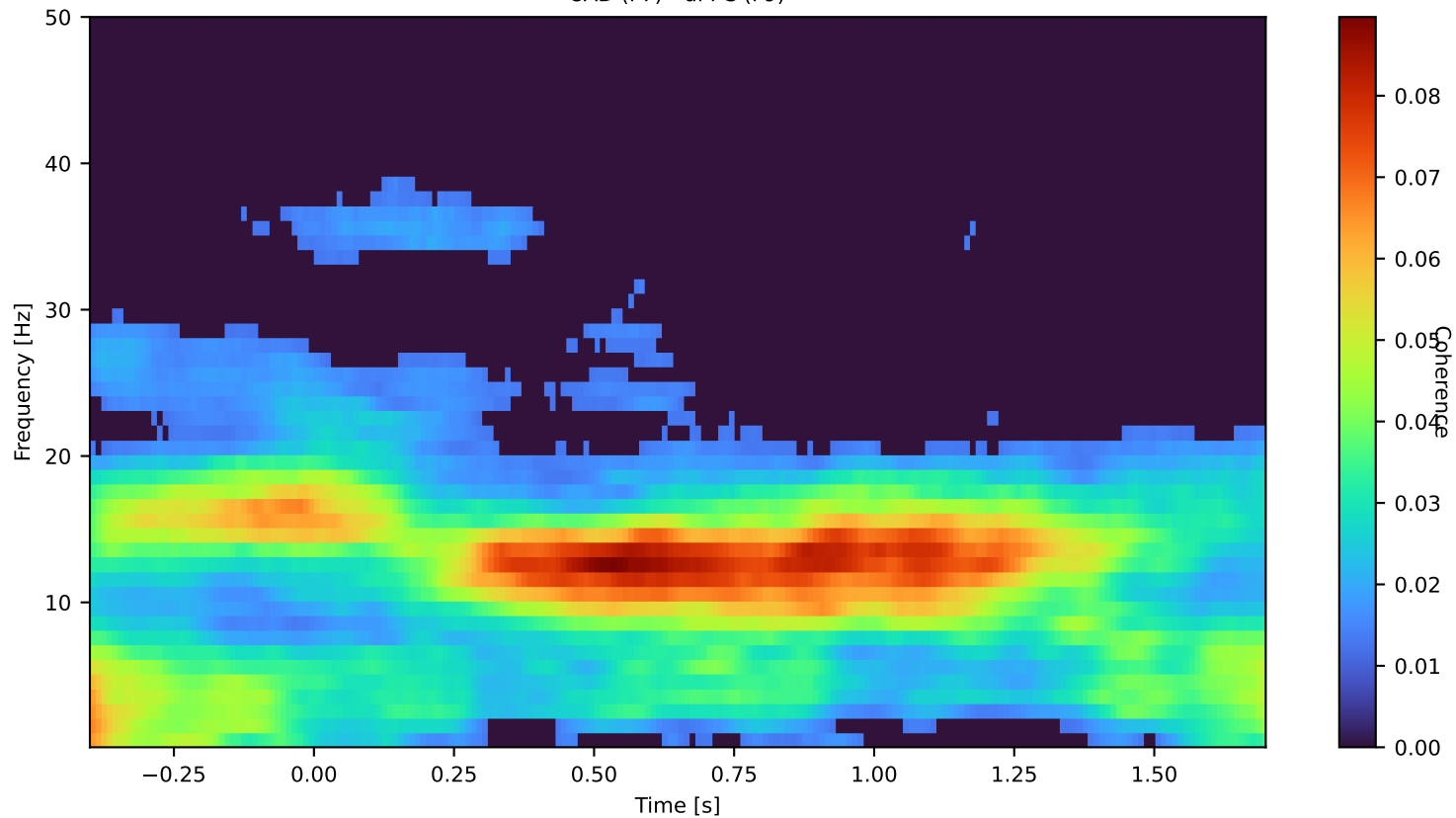
8AD (F7) - dPFC (F9)
